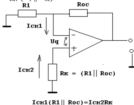
Рис. 14 Способ снижения величины тока смещения
