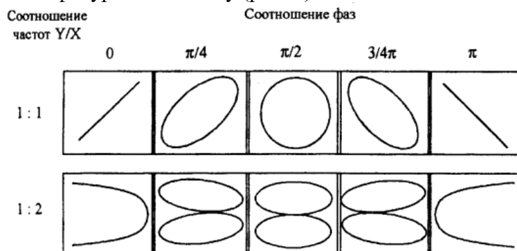
Рис. 5. Фигуры Лиссажу Генератор развертки.
