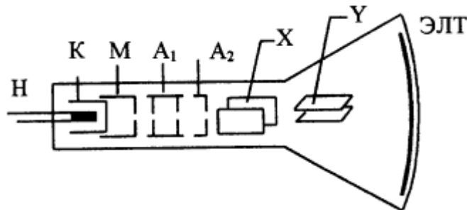
Рис. 2. Электронно-лучевая трубка
