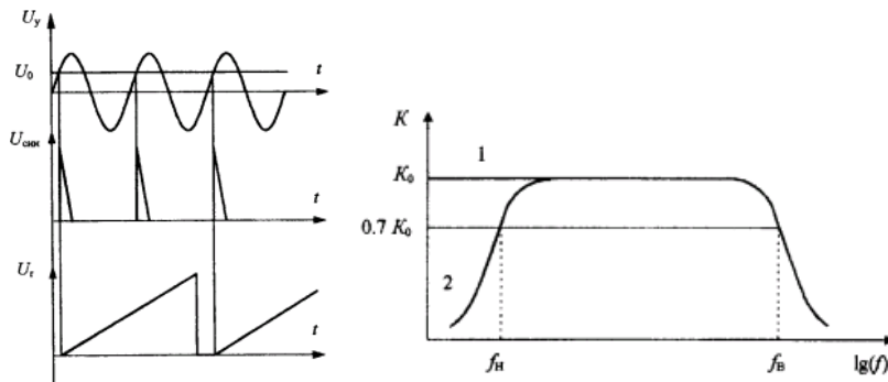
Рис. 8 Синхронизация генератора развертки: U_y - исследуемый сигнал, U_0 - уровень синхронизации, U_{\text{ан}} - синхрои́мпульс, U_r - напряжение развертки
