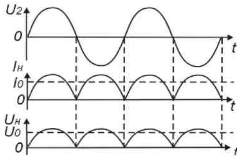
Рис. 6. Диаграммы напряжения и токов в мостовой схеме
