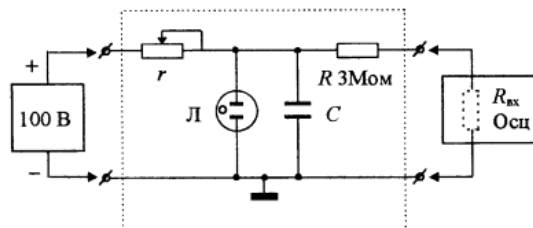
Рис. 13. Релаксационный генератор
